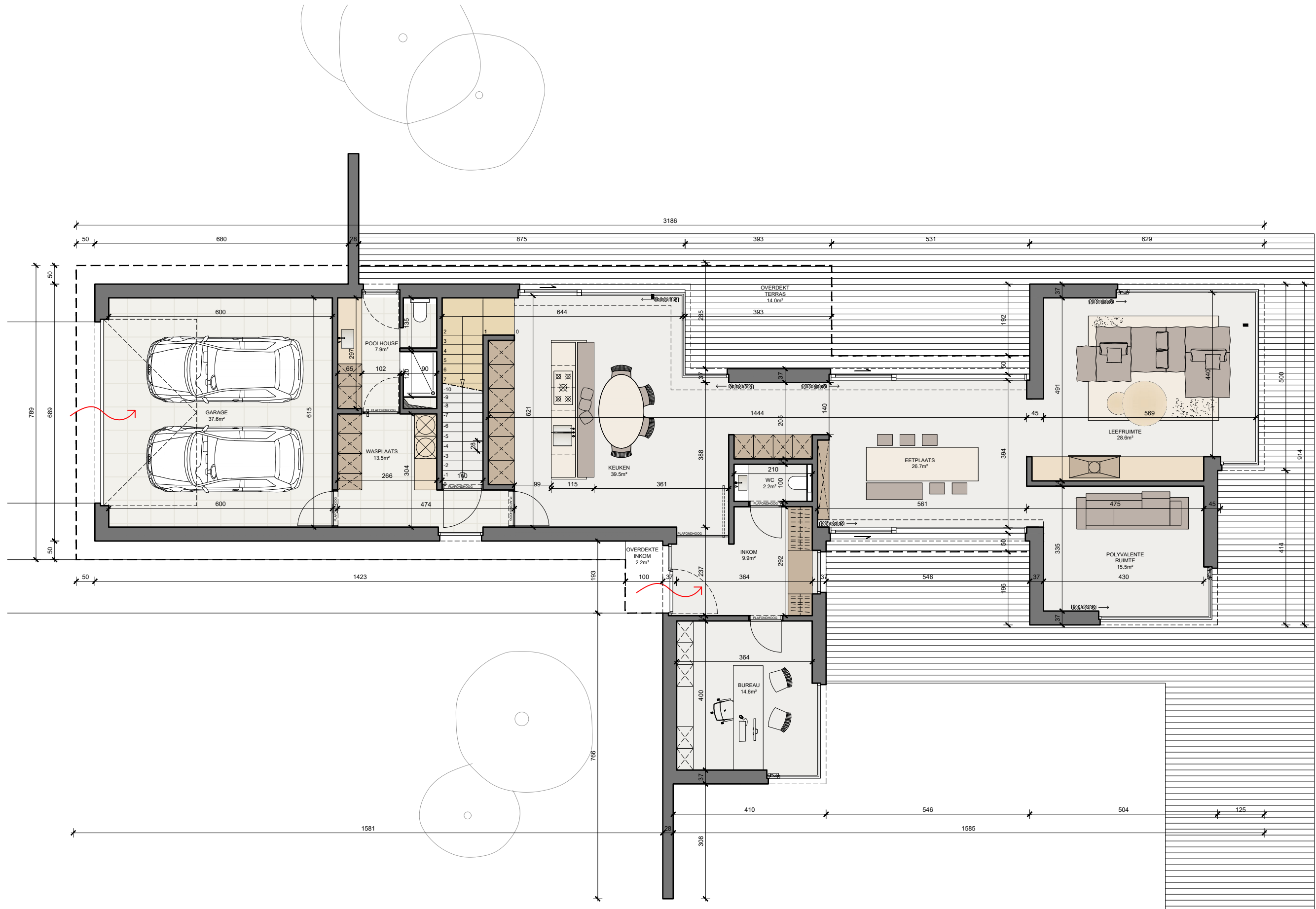
PLAN NIVEAU 0 WONING - BRUTO OPP. : 249.5m 2 incl. overdekt terras en overdekte inkom excl. luifels
